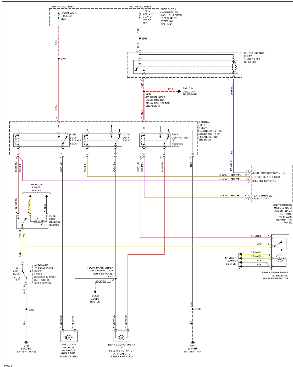
Fig. 47: Trunk, Tailgate, Fuel Door Circuits
