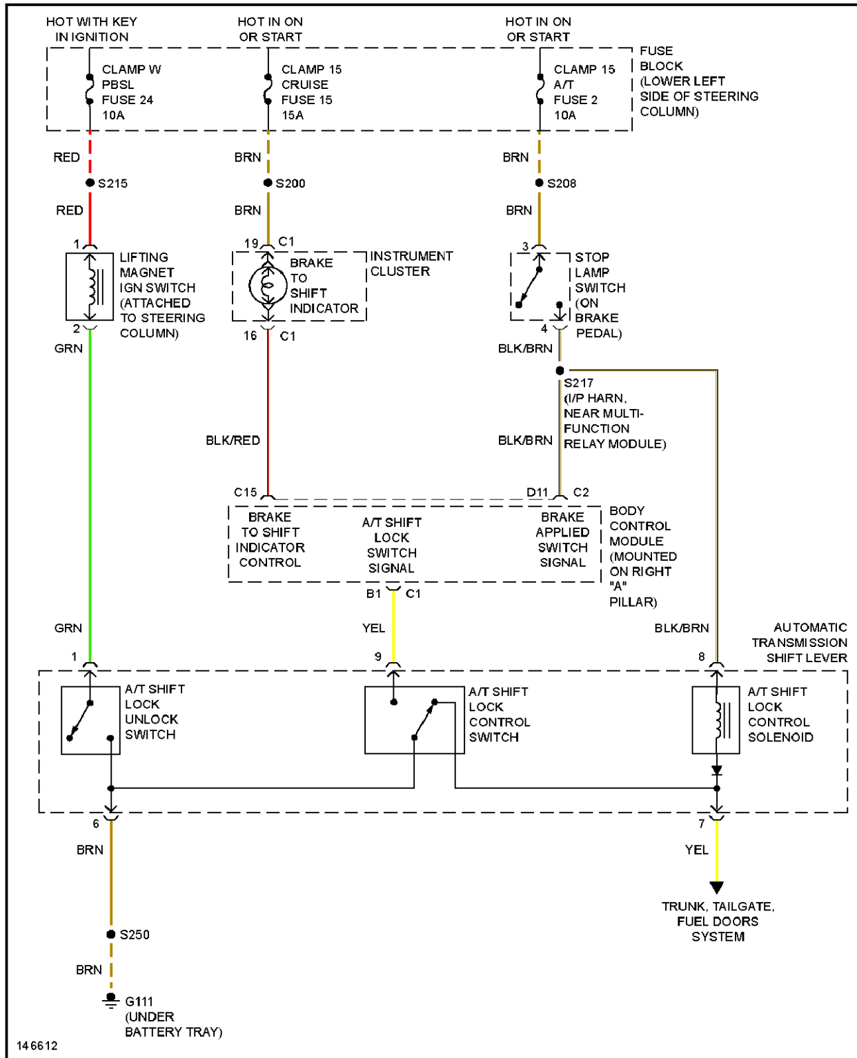
Fig. 42: Shift Interlock Circuit
